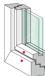
halbflächenversetzt
